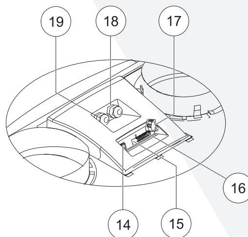
Pokrywa wyświetlacza - widok z tyłu
