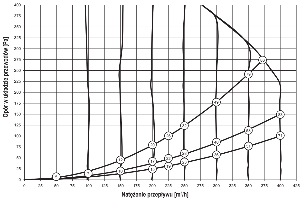
Charakterystyka wentylatora REQURA 400
