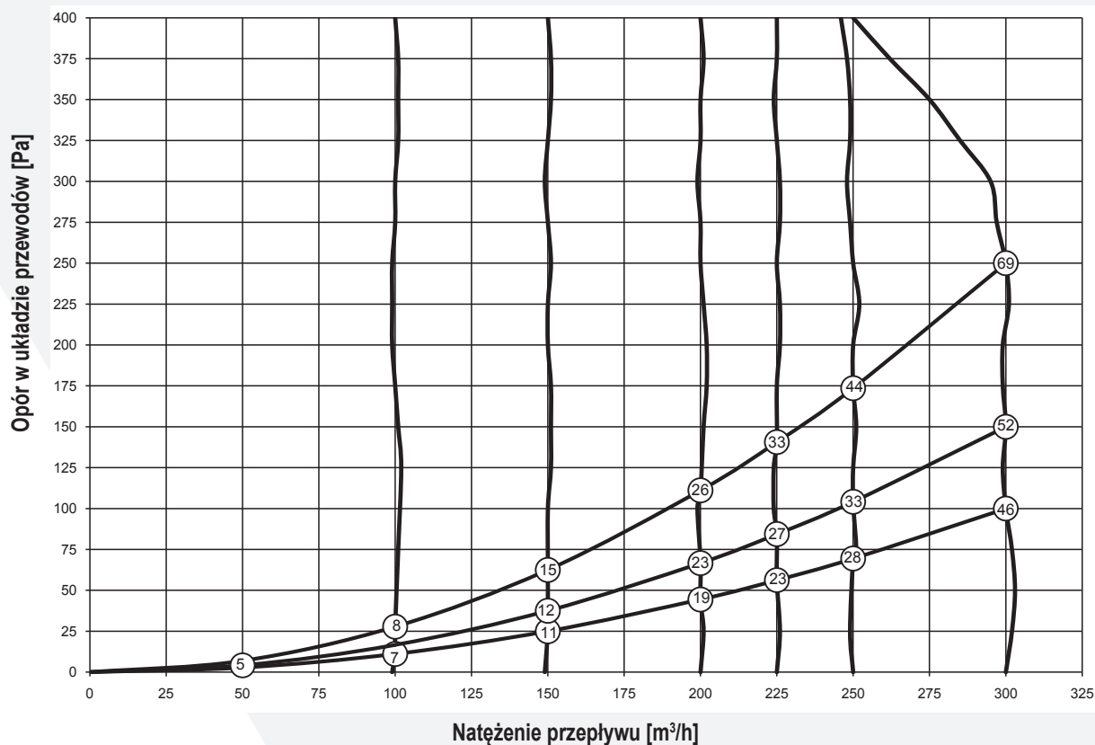
Charakterystyka wentylatora REQURA 300
