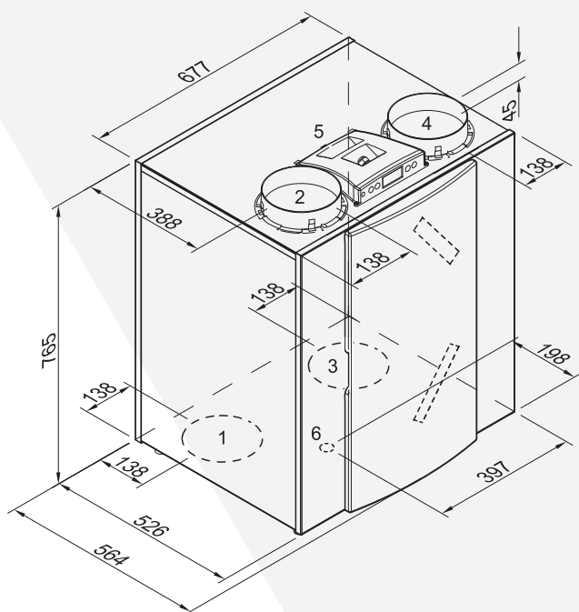
REQURA wersja prawa 2/2
