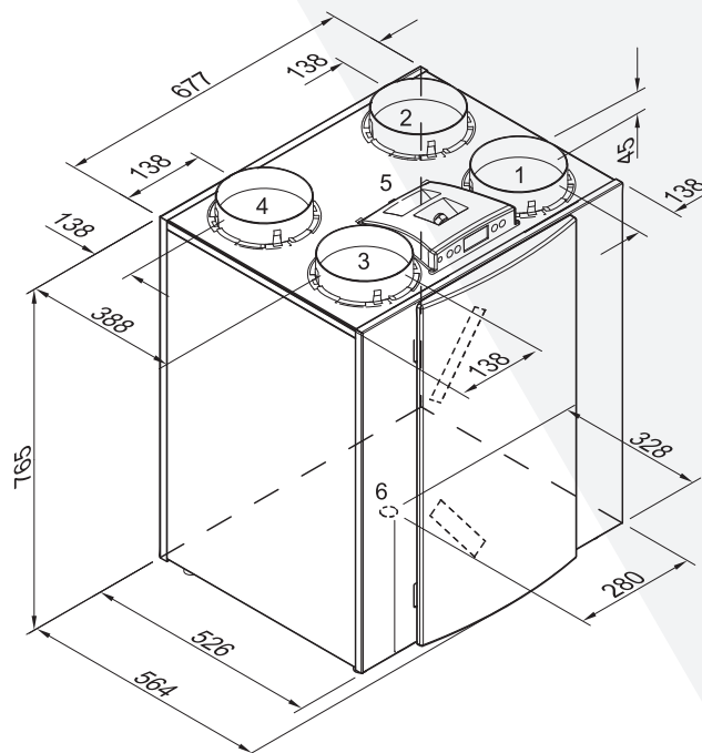
REQURA - wersja lewa 4/0
