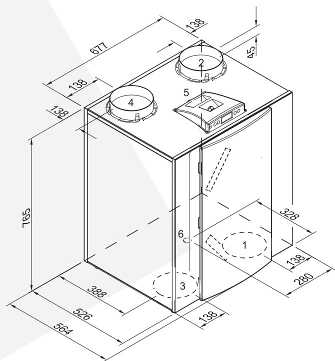
REQURA - wersja lewa 2/2
